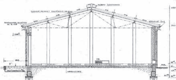
FIG.10 DOORSNEDE C-D
