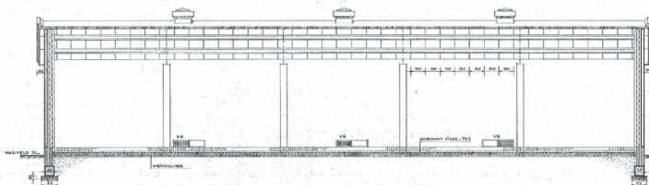
FIG.9 DOORSNEDE A-B
