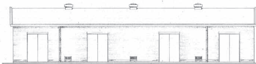
FIG.7 VOORGEVEL
